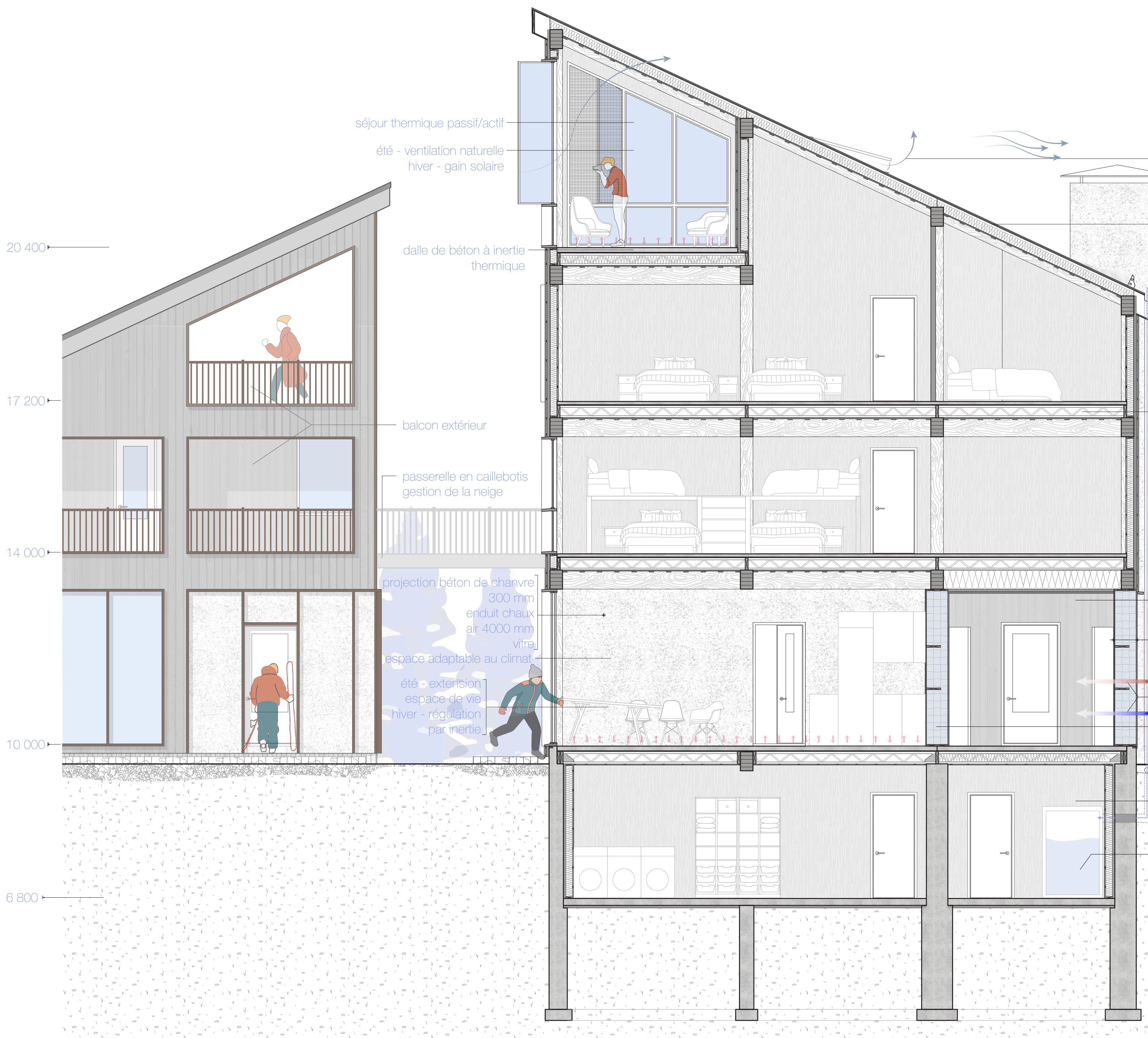
Coupes bioclimatiques
