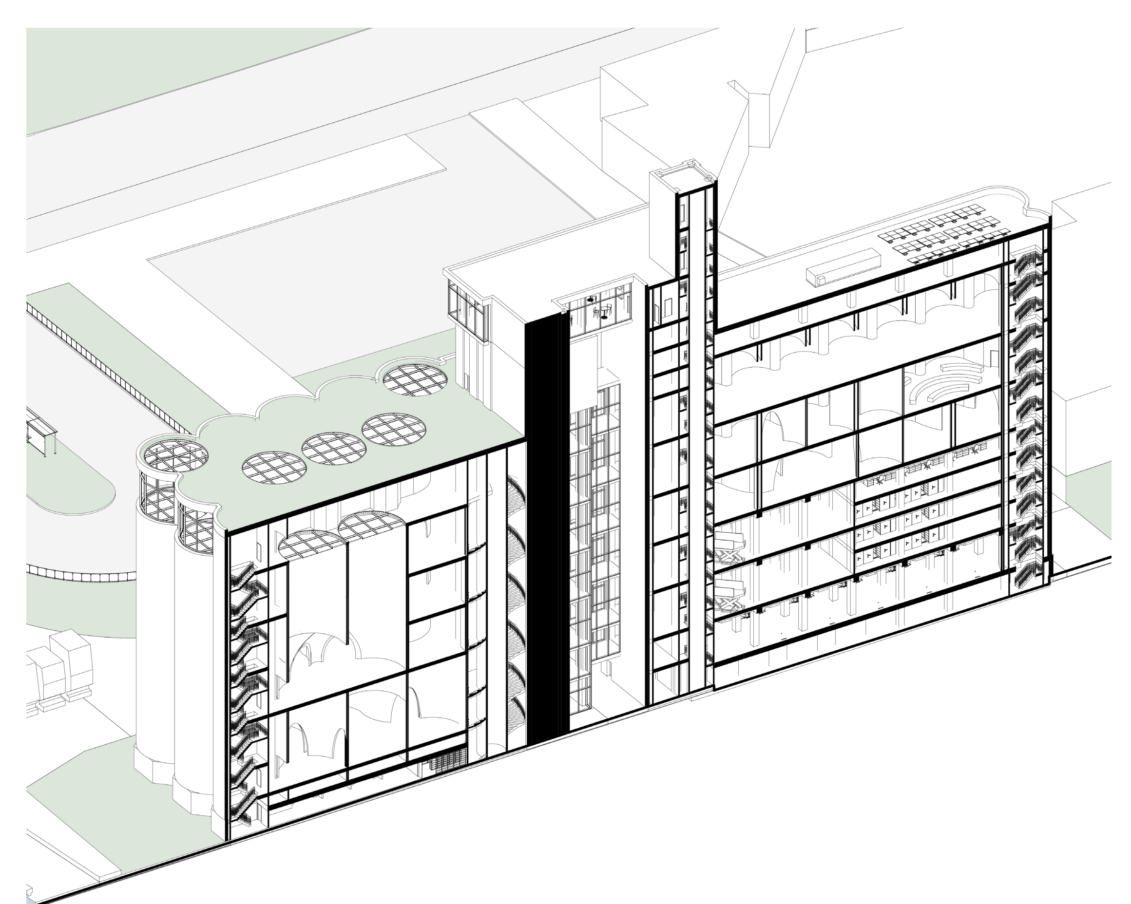
COUPE DANS LE BATIMENT - AXONOMETRIE COUPEE
