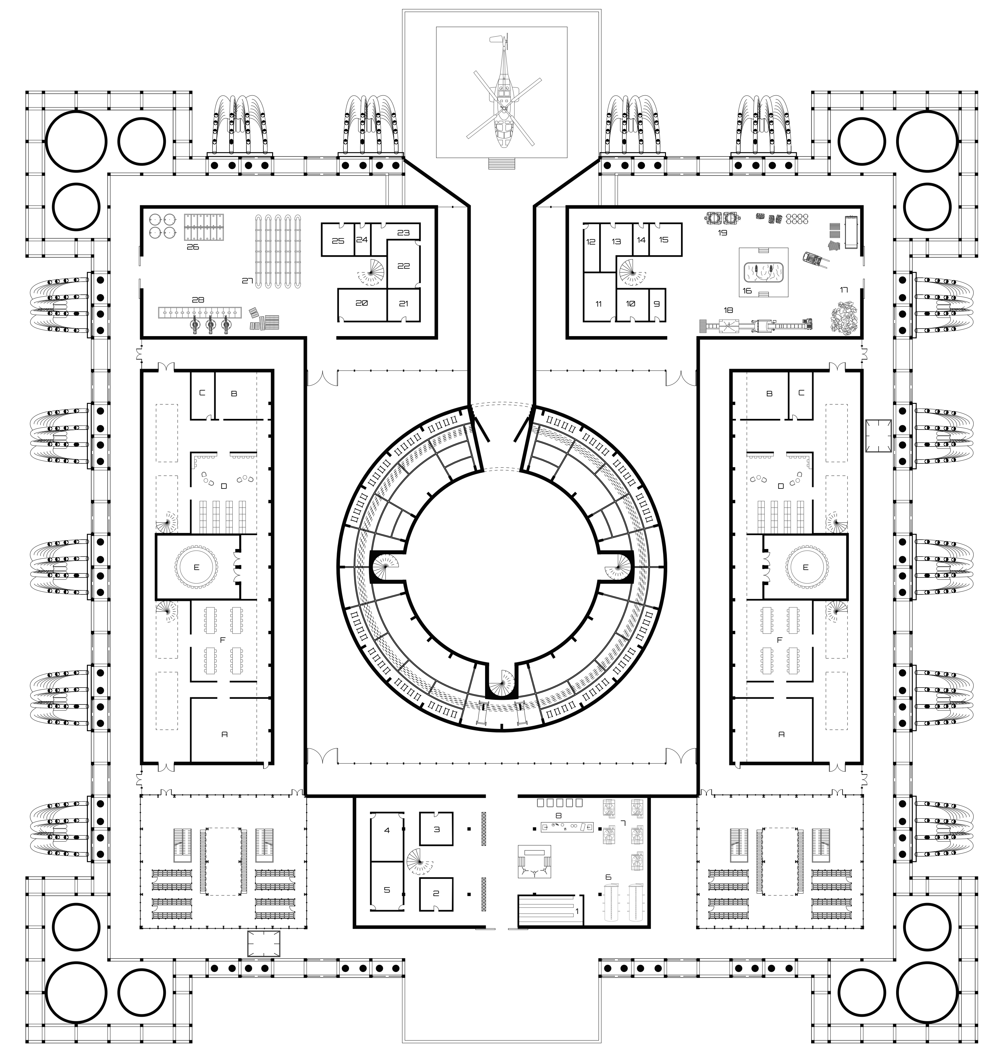
PLAN NIVEAU 0
