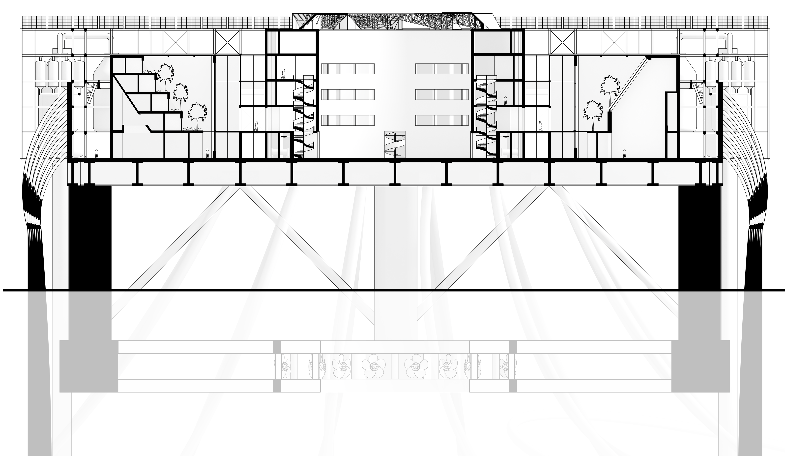
COUPE
